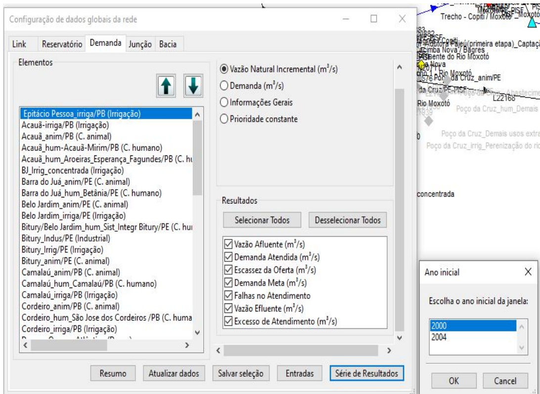
Figura 11.113 - Interface para configuração da tela de resultados no modo de simulações janelas para Demandas (Cenário de Clima).
