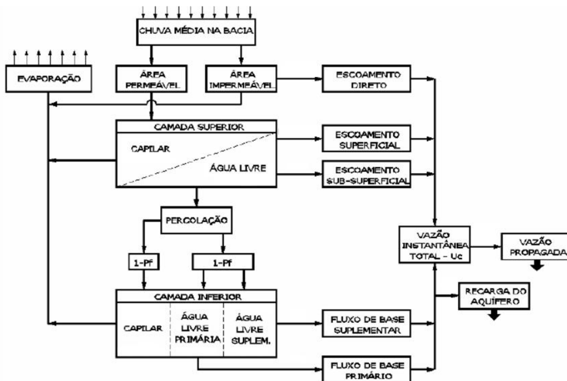
Figura 3.4 - Descrição do Modelo SACR.
