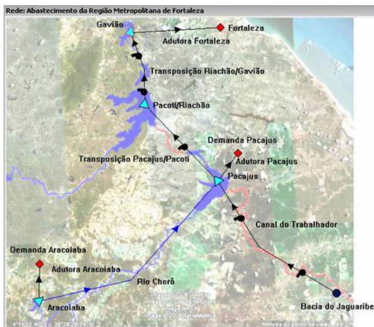
Figura 2.3 - Desenho esquemático do sistema de abastecimento da Região Metropolitana de Fortaleza no Ceará.
