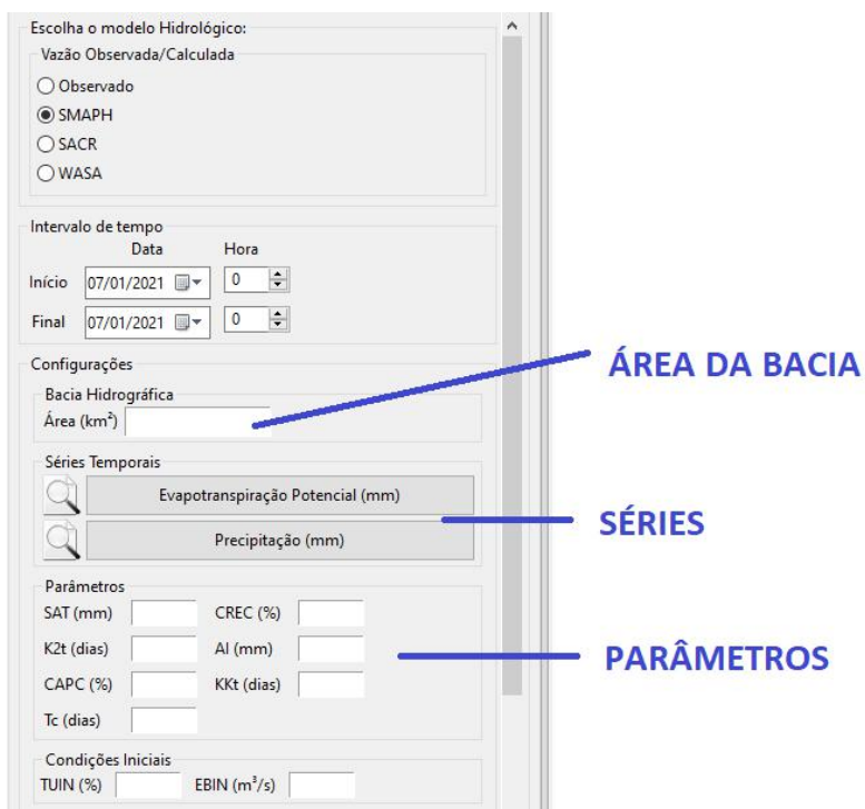
Figura 9.7 - Entrada de dados do modelo SMAP horário.
