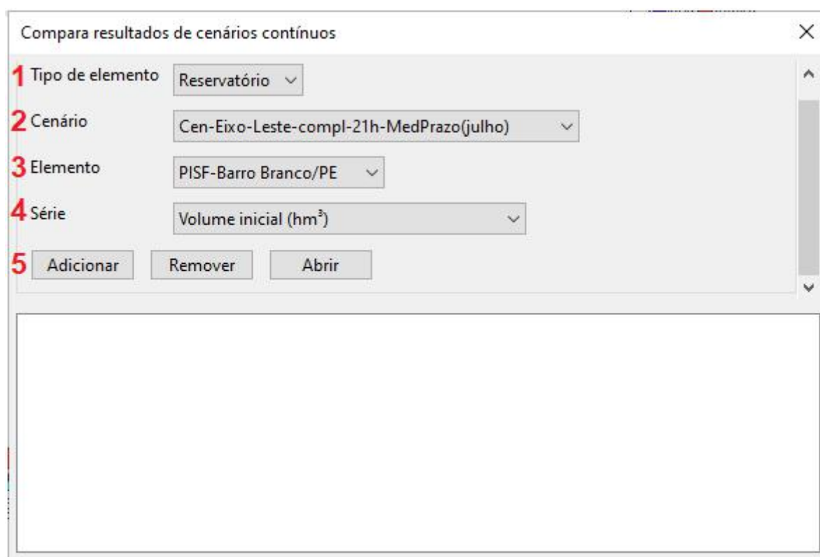
Figura 11.100 - Interface para seleção do(s) elemento(s) para comparação dos resultados (Método de Simulação Contínuo)
