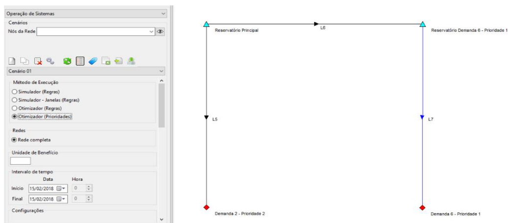
Figura B1.8 - Tela de exibição do arquivo importado.
