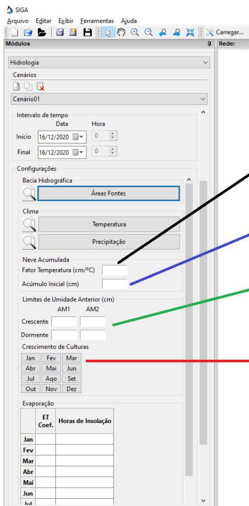
Figura 9.12 - Informações sobre balanço de acúmulo de neve e crescimento de culturas para simulação do modelo GWLF.
