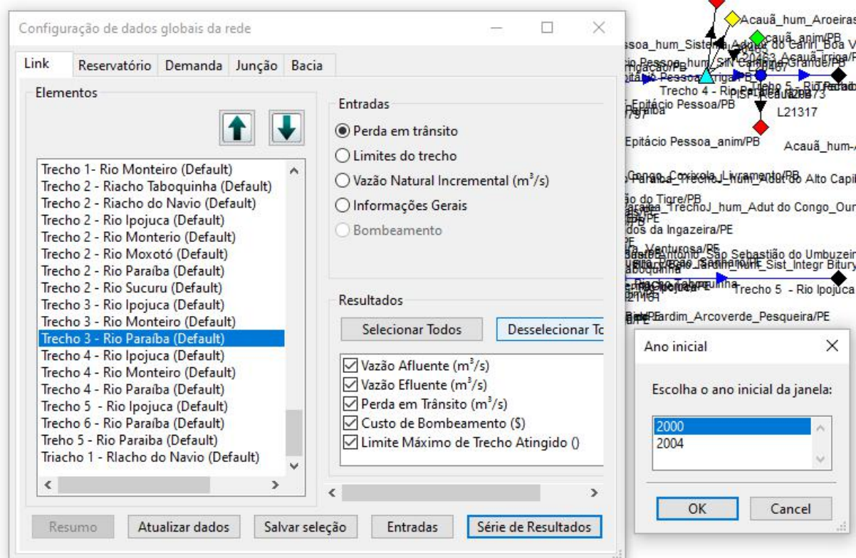
Figura 11.116 - Interface para configuração da tela de resultados no modo de simulações janelas para trecho/link (Cenário de Clima).
