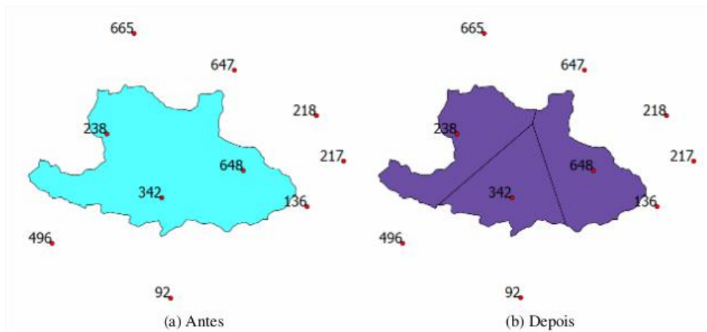
Figura C1.1 - Método de Thiessen/Voronoi
