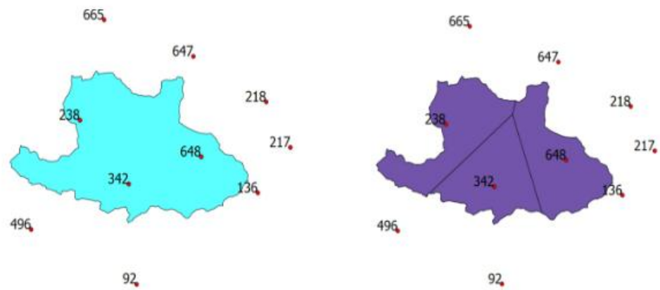
Figura 6.2 - Exemplo dos polígonos de Thiessen.
