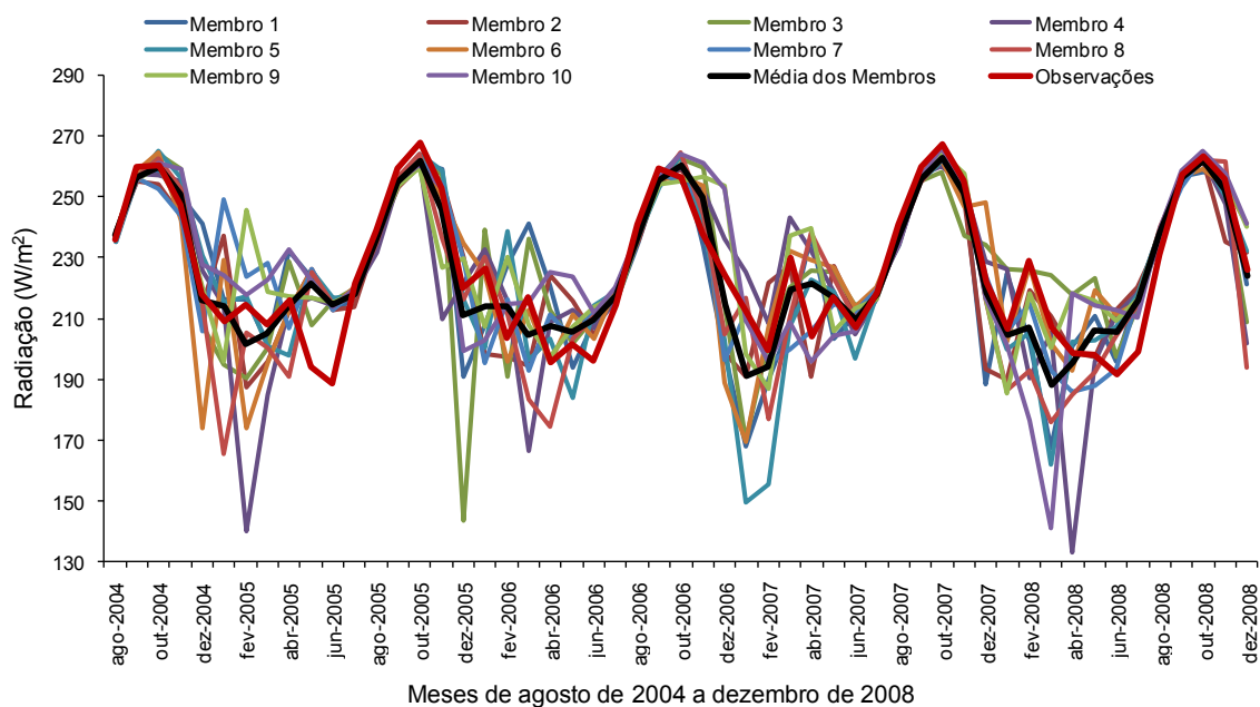
Figura 11. Radiação solar observada através das PCDs e através das simulações realizadas com o modelo RAMS para o período de agosto de 2004 a dezembro de 2008 após a aplicação da correção. Em vermelho, a radiação solar observada; em preto, a radiação média dos dez membros resultantes das simulações numéricas, mostradas pelas demais curvas coloridas.
