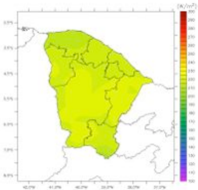
Figura 39. Climatologia da radiação solar ( \text{W/m}^2 ) para o quadrimestre FEV-MAR-ABR-MAI para anos SECOS.
