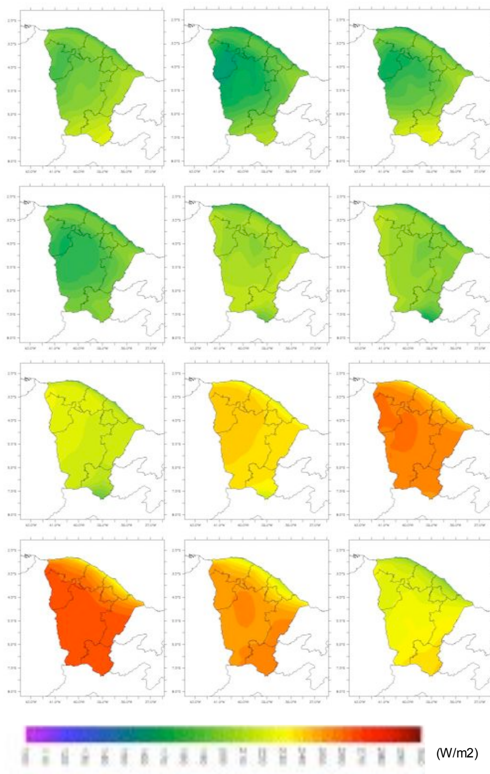
Figura 92. Média mensal da radiação solar ( \text{W/m}^2 ) para o ano de 2009.
