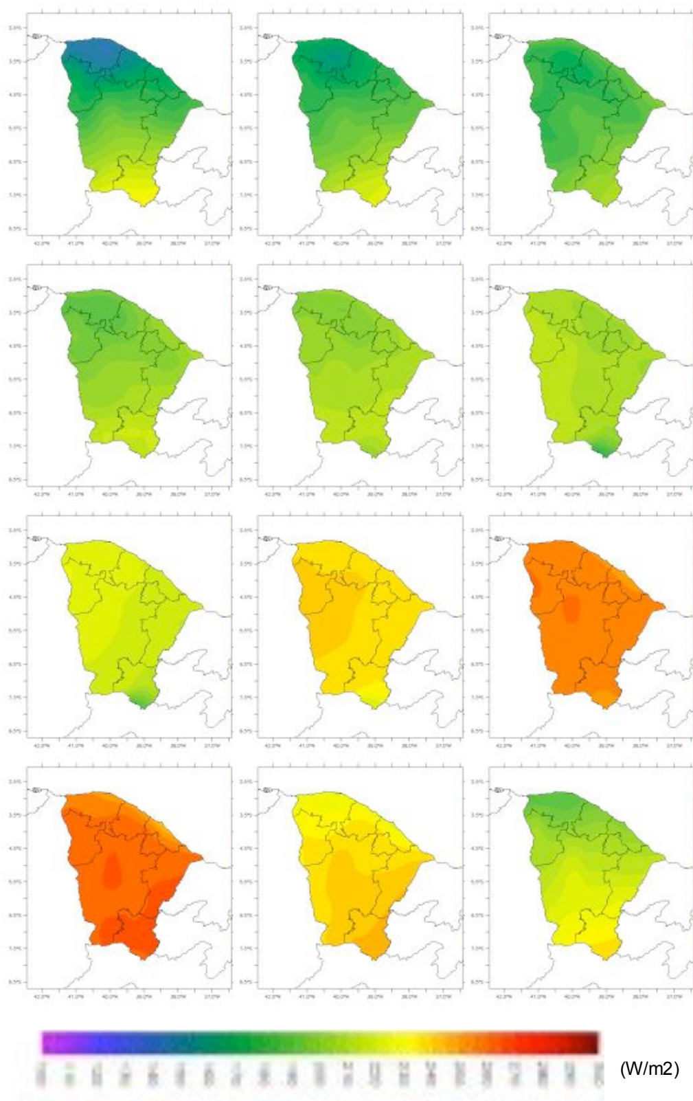
Figura 69. Média mensal da radiação solar (W/m 2 ) para o ano de 1986.
