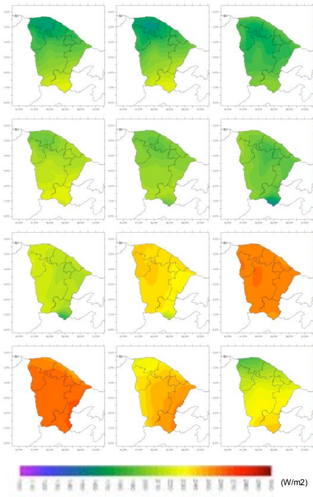
Figura 56. Média mensal da radiação solar ( \text{W/m}^2 ) para o ano de 1973.
