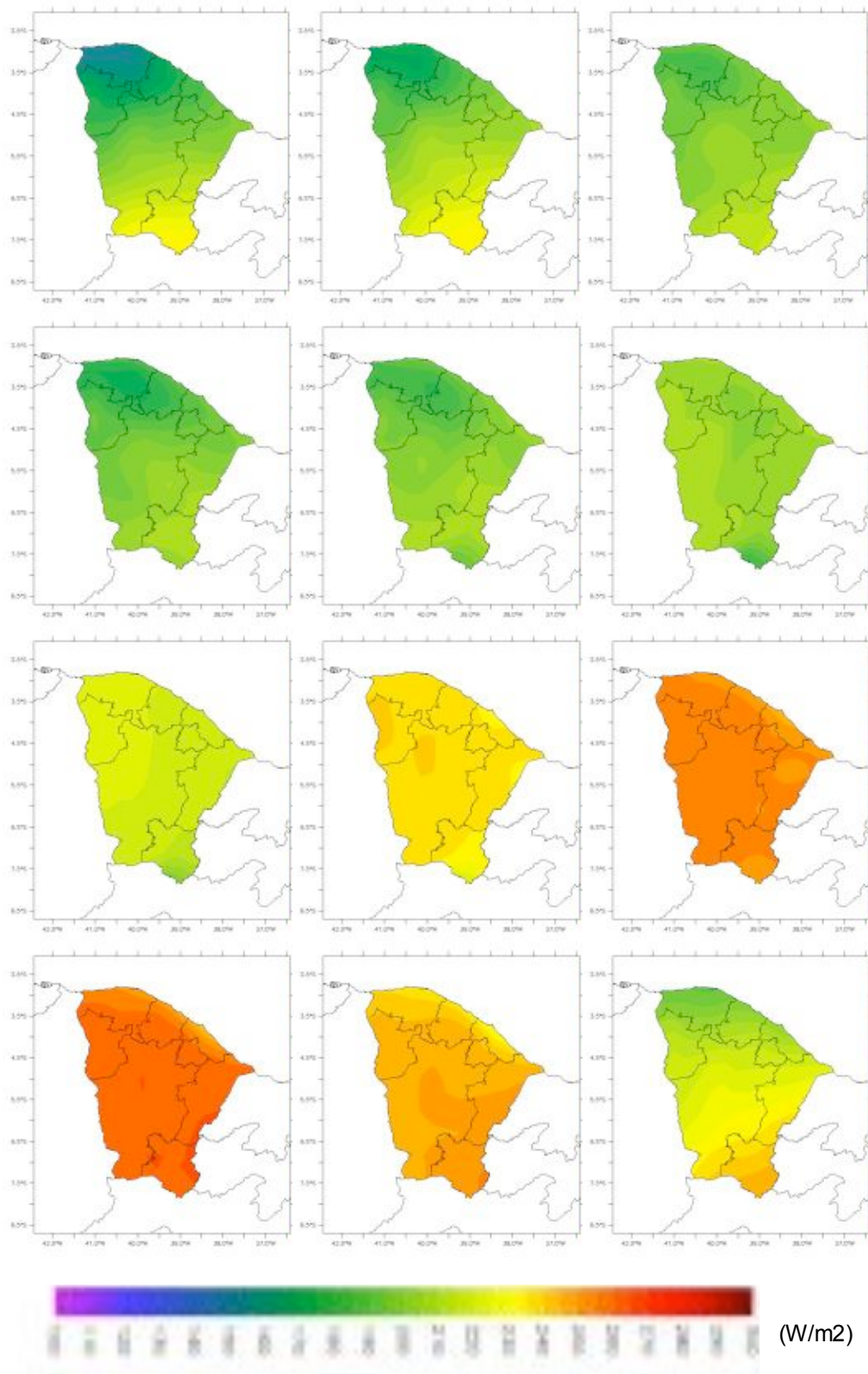
Figura 48. Média mensal da radiação solar ( \text{W/m}^2 ) para o ano de 1965.
