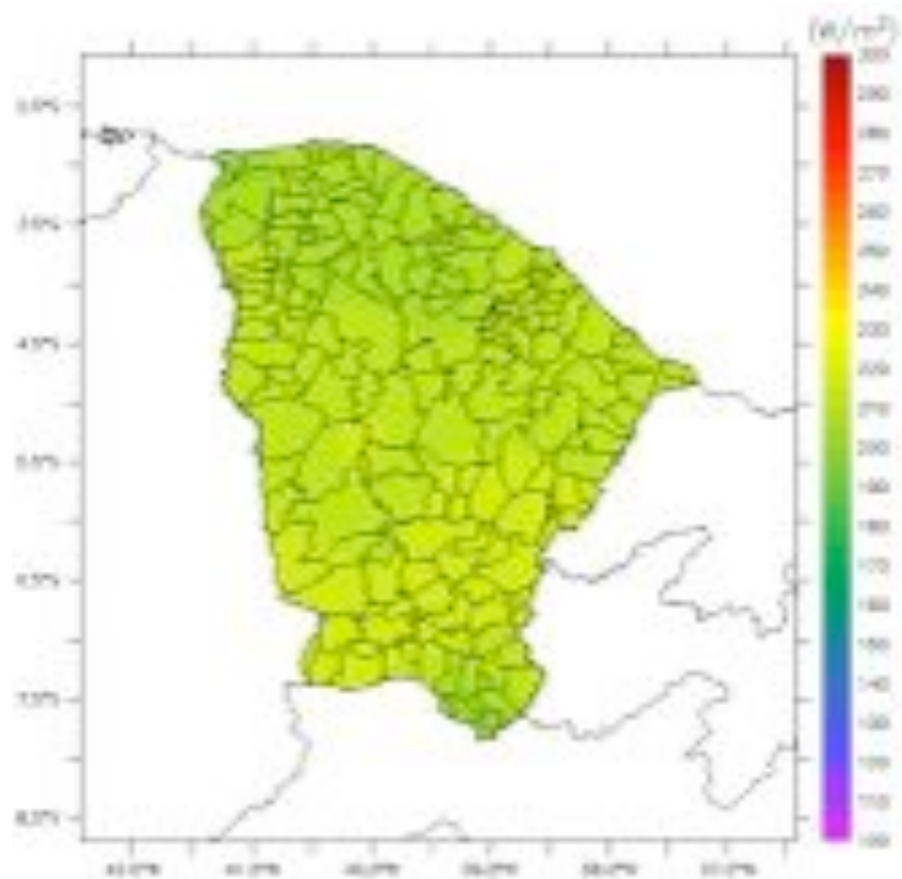
Figura 17. Climatologia da radiação solar ( \text{W/m}^2 ) para o mês de MAIO.
