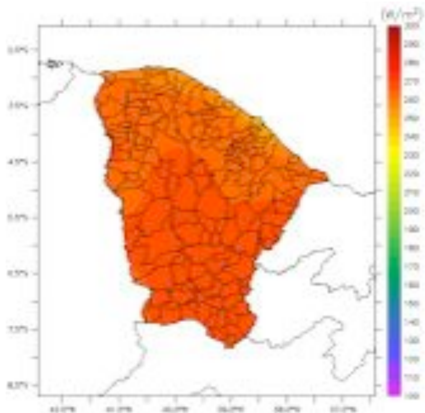
Figura 22. Climatologia da radiação solar ( W/m^2 ) para o mês de OUTUBRO.
