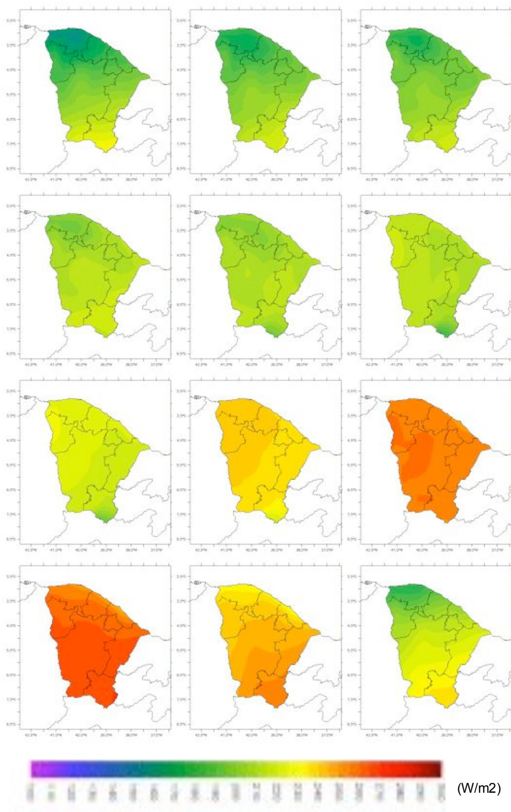
Figura 60. Média mensal da radiação solar ( \text{W/m}^2 ) para o ano de 1977.
