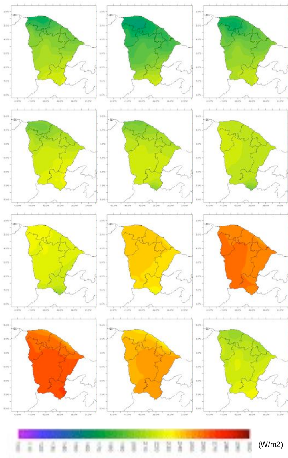
Figura 74. Média mensal da radiação solar ( \text{W/m}^2 ) para o ano de 1991.
