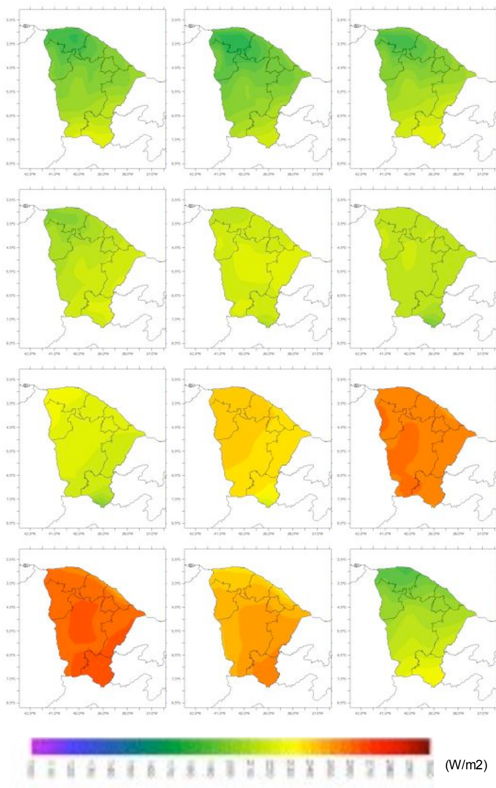
Figura 70. Média mensal da radiação solar ( \text{W/m}^2 ) para o ano de 1987.
