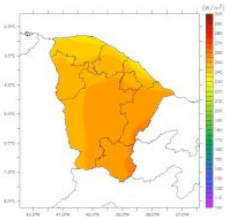
Figura 40. Climatologia da radiação solar ( W/m^2 ) para o semestre JUN-JUL-AGO-SET-OUT-NOV para anos NORMAIS.
