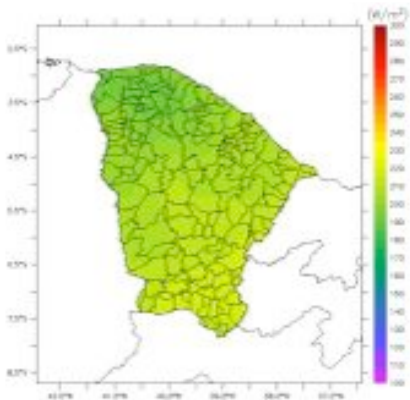
Figura 16. Climatologia da radiação solar ( \text{W/m}^2 ) para o mês de ABRIL.
